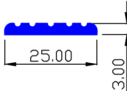
MAAN SEC.-90234 0.177 Kg/Mtr.
