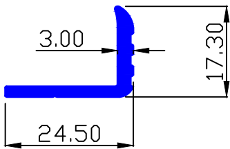
MAAN SEC.-90188 0.236 Kg/Mtr.
