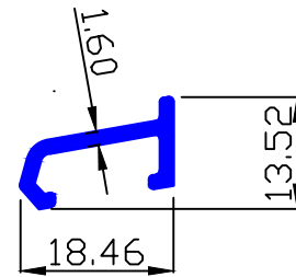
MAAN SEC.-90252 0.154 Kg/Mtr.
