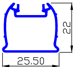
MAAN SEC.-91070 0.226 Kg/Mtr.
