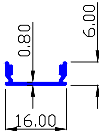
MAAN SEC.-91070 0.226 Kg/Mtr.
